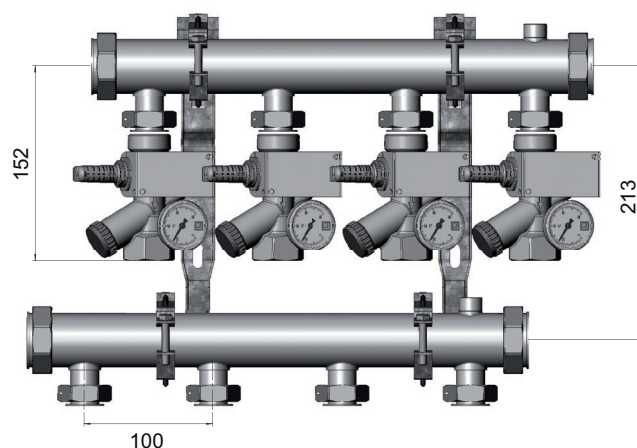
Installationsexempel mot LK Fördelare Qmax G40 som grupp-fördelare eller som markvärme-fördelare.
