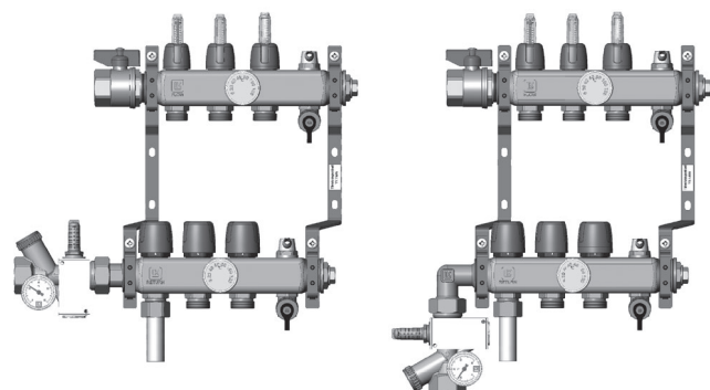
Installationsexempel mot LK Värmekrets-fördelare RF i rakt resp. vinklat utförande.
