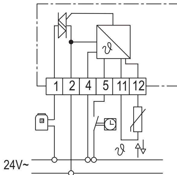
Kopplingsschema för LK Rumstermostat S2 EXT (Kopplingsschema för LK Rumstermostat S2 är lika men saknar plint 11 och 12 för extern givare)
